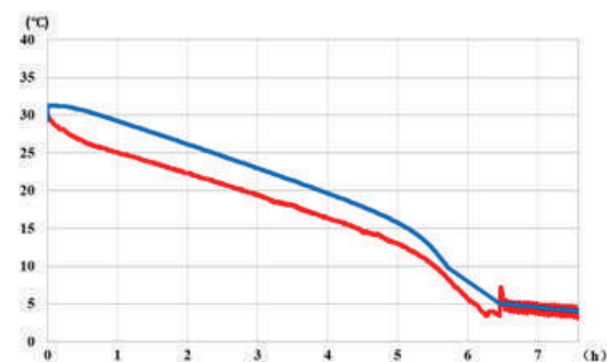
Variazione della temperatura dell'acqua nel contenitore, mentre la temperatura ambiente è di di -35^{\circ}C , con un carico superficiale di 0.1 W/cm^2 (300W). Si può notare che, nonostante l'aumento della potenza di riscaldamento, la temperatura interna del serbatoio continua a scendere lentamente.
