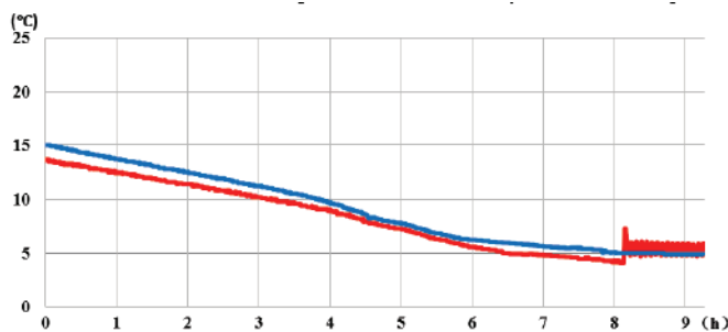
Variazione della temperatura dell'acqua nel contenitore, mentre la temperatura ambiente è di -10^{\circ}C , con un carico superficiale di 0.05 W/cm^2 (150W). Si può notare che la temperatura interna del contenitore si stabilizza a 5^{\circ}C .
