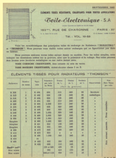
Tessuto riscaldante in amianto (1960 Toile-électronique, Ultimheat Museum)
