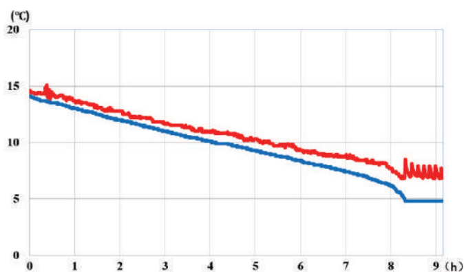
Variazione della temperatura dell'acqua nel contenitore, mentre la temperatura ambiente è di -10^{\circ}\text{C} , con un carico superficiale di 0.05 \text{ W/cm}^2 (150W). Si può notare che la temperatura interna del contenitore si stabilizza a 5^{\circ}\text{C} .
