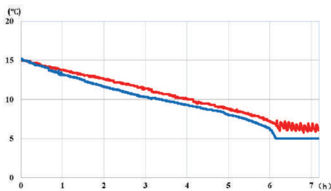
Variazione della temperatura dell'acqua nel contenitore, mentre la temperatura ambiente è di -15^{\circ}\text{C} , con un carico superficiale di 0.05 \text{ W/cm}^2 (150W). Si può notare che la temperatura interna del contenitore si stabilizza a 5^{\circ}\text{C} .
