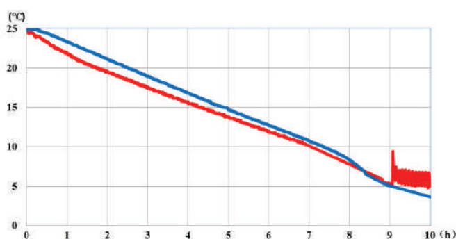
Variazione della temperatura dell'acqua nel contenitore, mentre la temperatura ambiente è di -20^{\circ}\text{C} , con un carico superficiale di 0.05 \text{ W/cm}^2 (150W). Si può notare che la temperatura interna del serbatoio continua a scendere nettamente.
