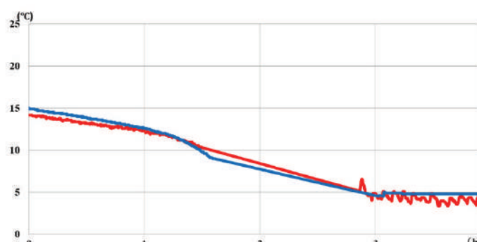
Variazione della temperatura dell'acqua nel contenitore, mentre la temperatura ambiente è di -35^{\circ}\text{C} , con un carico superficiale di 0.1 \text{ W/cm}^2 (150W). Si può notare che l'aumento di potenza permette di stabilizzare la temperatura interna del contenitore a 5^{\circ}\text{C} .
